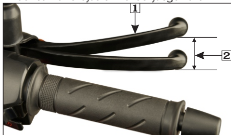
(1) Palanca freno delantero (2) Juego libre 10-20 mm
