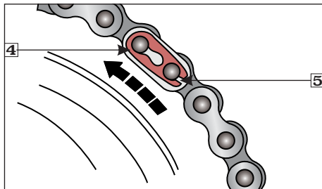
(4) Placa de bloqueo
