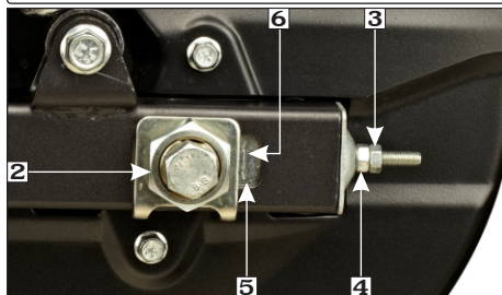
(2) Tuerca del mango (3) Tuerca de bloqueo (4) Tuerca de ajuste (5) Marca índice (6) Borde trasero de la ranura de ajuste
