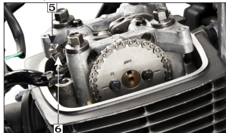
(5) Tornillo de ajuste (6) Tuerca de bloqueo
