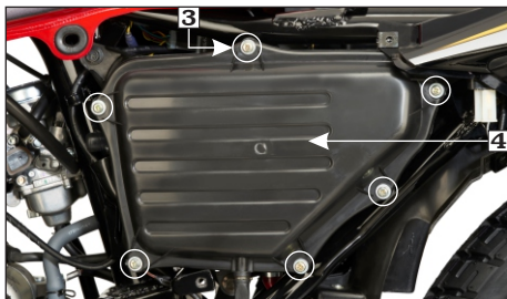
(3) Tornillos cubierta filtro de aire (4) Cubierta filtro de aire
