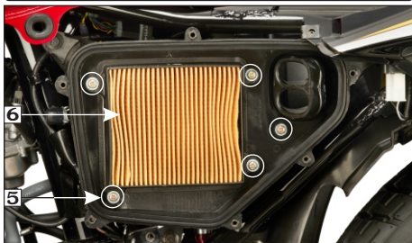
(5) Tornillos del elemento filtro de aire (6) Elemento filtro de aire
