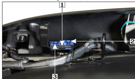
(1) Portafusible (2) Fusible 15A (3) Fusible de repuesto 15A
